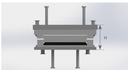
Schnitt durch TE Lager ohne Ankerplatten mit Dollen
