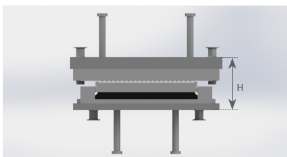
Schnitt durch TA Lager ohne Ankerplatten mit Gewindehülsen
